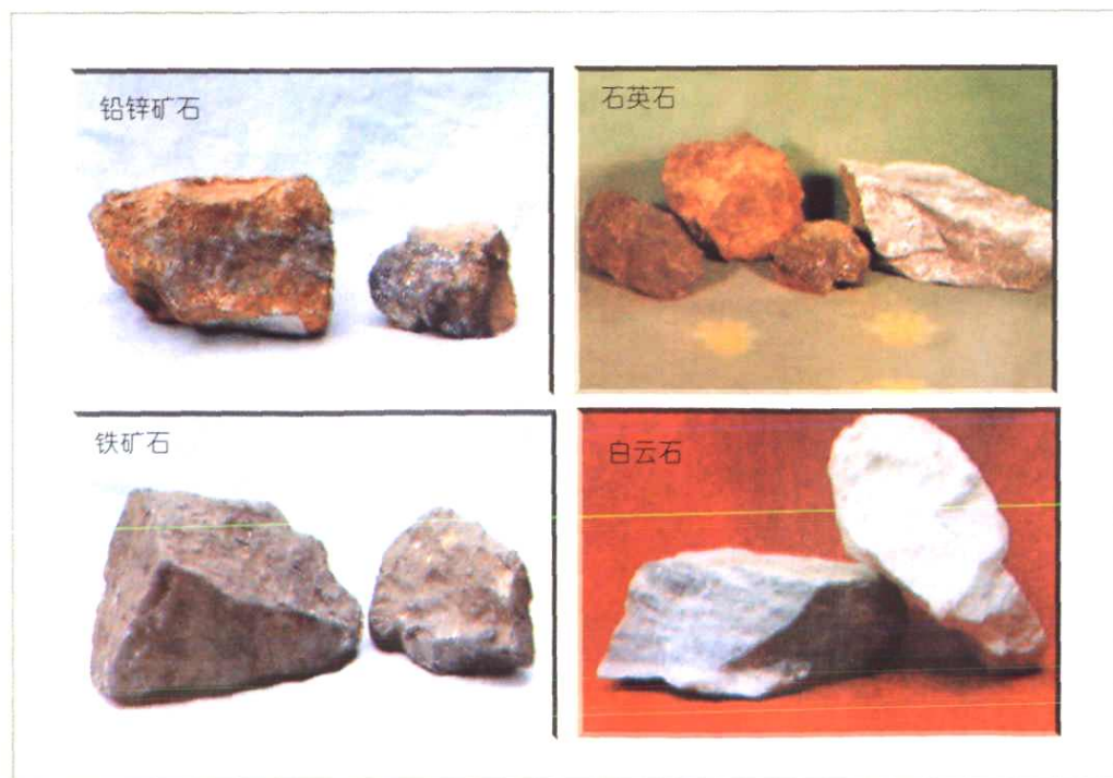
矿石标本
