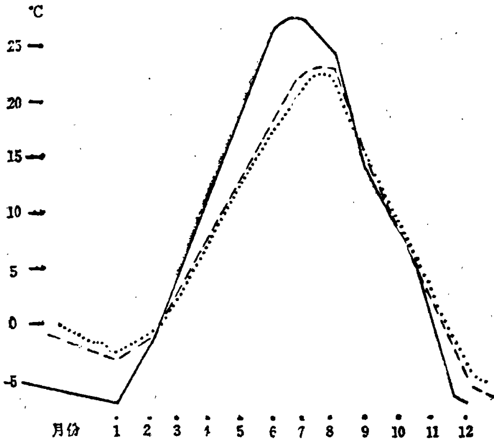
图例：月平均地面温度——月平均10cm地温·····月平均20cm地温·····
