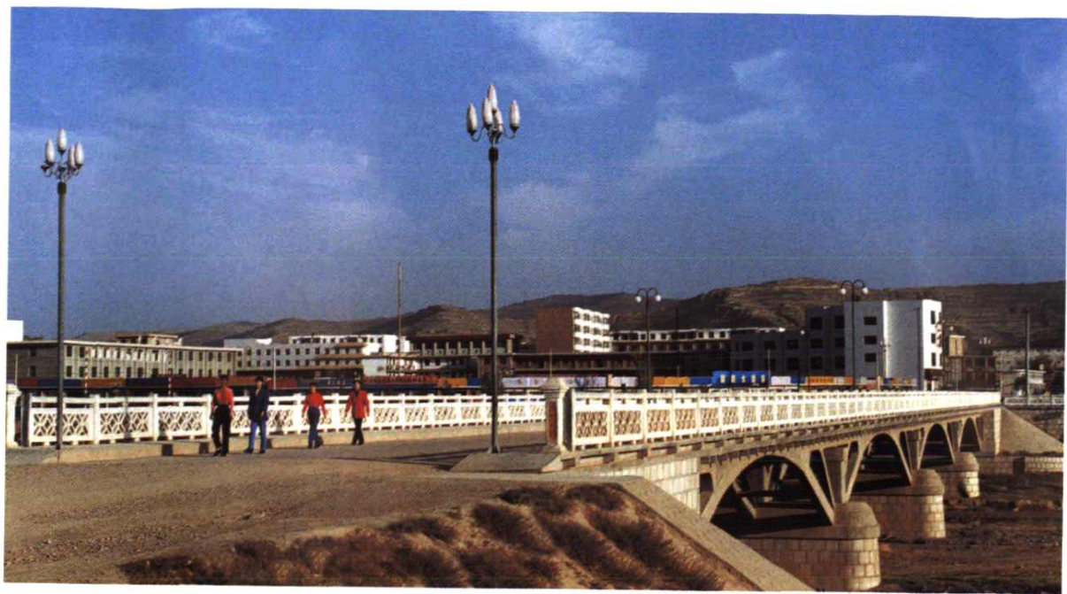
何马大桥
