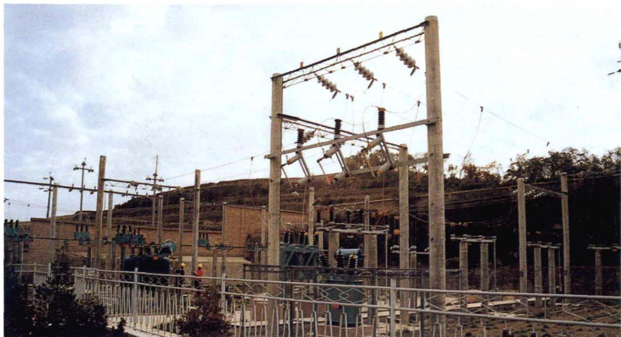
卧龙变电站
