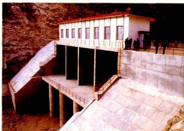
鞍子山拦河闸
