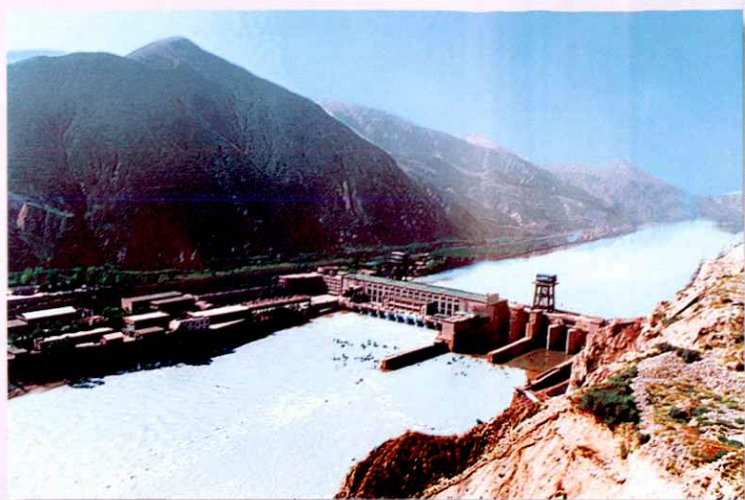
八盘峡水电厂
