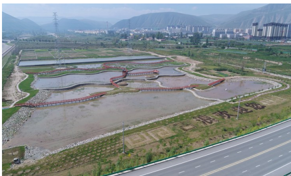
古浪县城区生活污水处理厂尾水人工湿地水质净化工程
