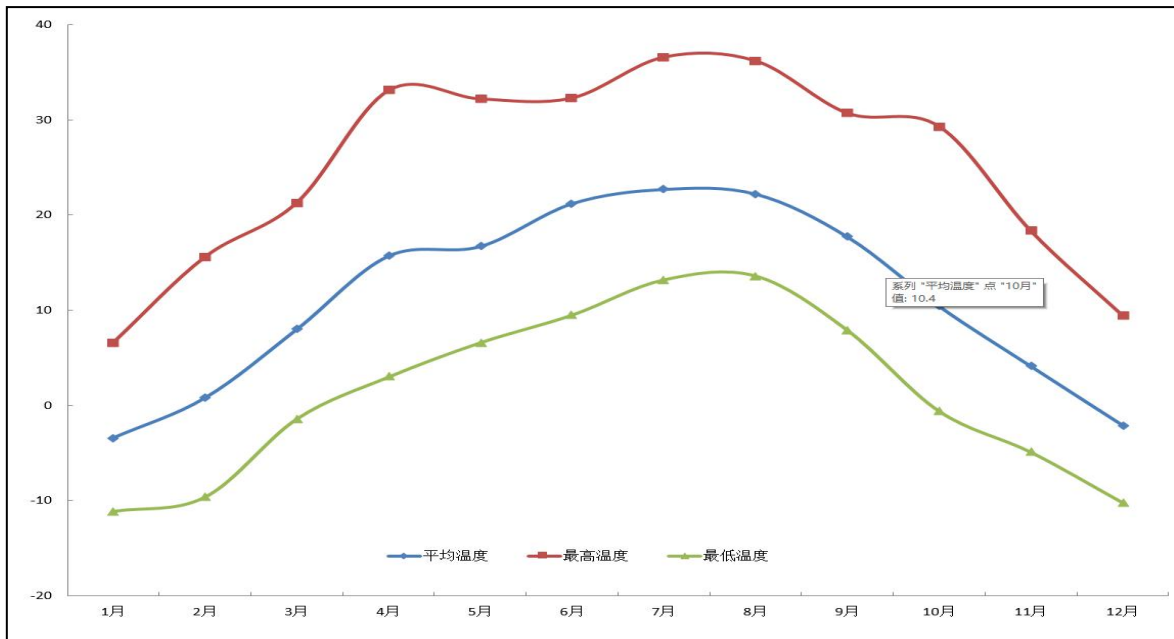
2019 年城关区各月气温分布图
