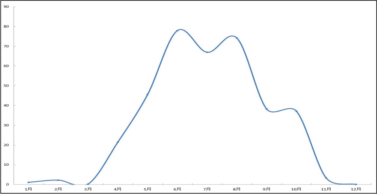
2019 年城关区各月降水分布
