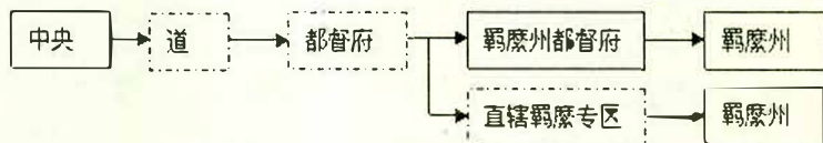
唐羁縻州政区的类型与管理层级示意图(点划线表示准政区,虚线表示地理区)
