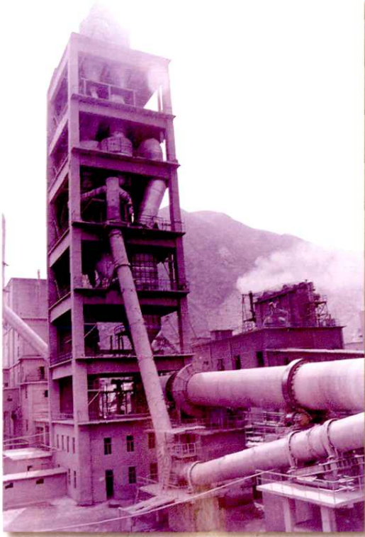
兰州市窑街水泥厂旋窑分解炉
