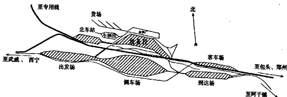
图 2 兰州西编组站示意图
