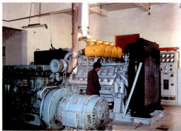
油机发电机组(1993年摄)
