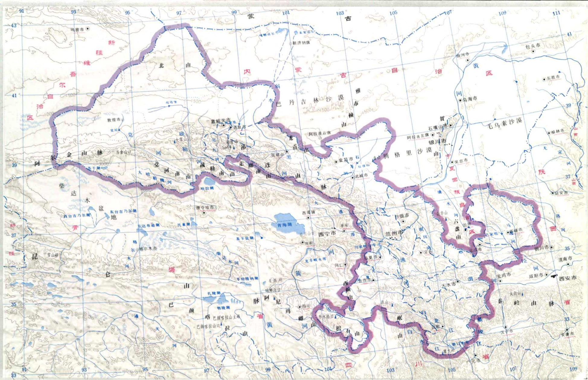
甘肃地势 1:700万
